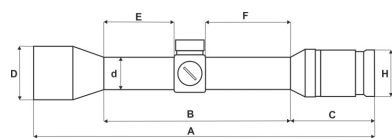
Rozměry E a F udávají ideální prostor pro uchytcení montáže
